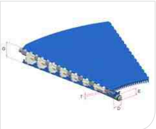
Type 型号 : HS-2000A-GB Pitch 节距 : -- Thickness 厚度 : 10MM Open area 开孔率 : 0%
