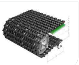
Type 型号 : HS-2600B Pitch 节距 : 25MM Thickness 厚度 : 11MM Open area 开孔率 : 44%
