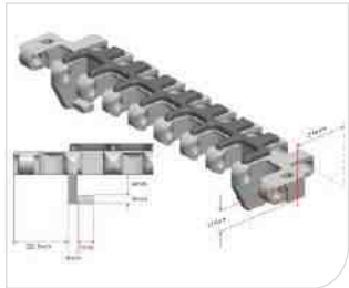
Type 型号：HS-500B-EL-GB Pitch 节距：25MM Thickness 厚度：15.5MM Open area 开孔率：36%
