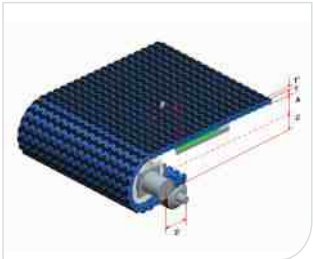
Type 型号 : HS-1500EL Pitch 节距 : 12.7MM Thickness 厚度 : 11MM Open area 开孔率 : 0%
