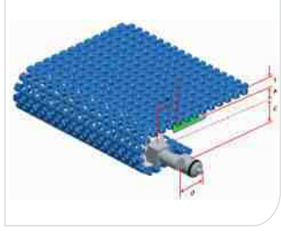
Type 型号：HS-500B-HD Pitch 节距：25MM Thickness 厚度：12.7MM Open area 开孔率：38%
