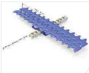
Type 型号 : HS-2200B1 Pitch 节距 : 19.05MM Width 宽度 : 400MM,600MM Open area 开孔率 : --
