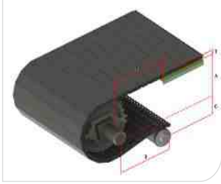
Type 型号 : HS-F1000A-N Pitch 节距 : 25.4MM Thickness 厚度 : 8.6MM Open area 开孔率 : 0%
