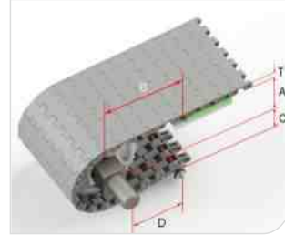
Type 型号 : HS-3400A Pitch 节距 : 25.4MM Thickness 厚度 : 12.8MM Open area 开孔率 : 0%
