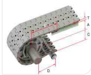
Type 型号 : HS-1000AB-76 Pitch 节距 : 19MM Thickness 厚度 : 8.5MM Open area 开孔率 : 2%
