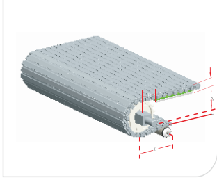
Type 型号：HS-500A-N Pitch 节距：25MM Thickness 厚度：16.4MM Open area 开孔率：0%
