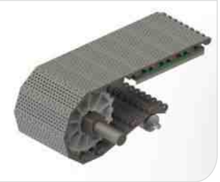
Type 型号：HS-101B-HD Pitch 节距：50.8MM Thickness 厚度：16MM Open area 开孔率：17.1%
