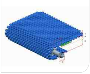
Type 型号：HS-500B-HD-D Pitch 节距：25MM Thickness 厚度：21.7MM Open area 开孔率：36%
