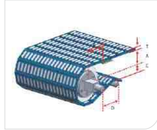
Type 型号 : HS-3800-6C Pitch 节距 : 80.80MM Thickness 厚度 : 13MM Open area 开孔率 : 0%
