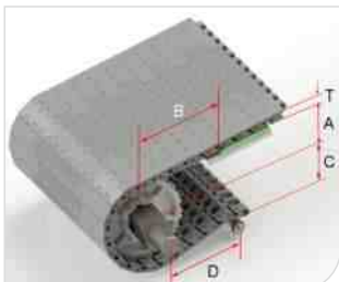
Type 型号 : HS-3400ZS Pitch 节距 : 25.4MM Thickness 厚度 : 12.8MM Open area 开孔率 : 0%
