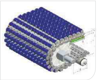
Type 型号：HS-600C Pitch 节距：25.4MM Thickness 厚度：32MM Open area 开孔率：36%
