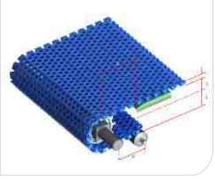
Type 型号：HS-500B-N Pitch 节距：25MM Thickness 厚度：12.7MM Open area 开孔率：35%
