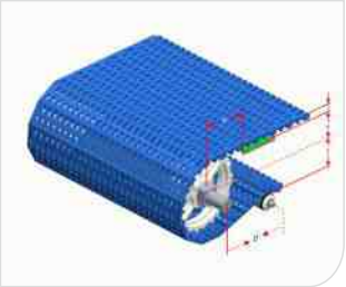
Type 型号：HS-103B-HD Pitch 节距：50.8MM Thickness 厚度：16MM Open area 开孔率：22%
