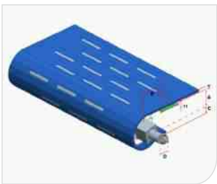
Type 型号 : HS-4800A-EL Pitch 节距 : 25.4MM Thickness 厚度 : 13.5MM Open area 开孔率 : 0%
