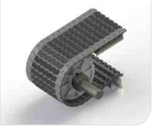
Type 型号 : HS-1000EL Pitch 节距 : 19MM Thickness 厚度 : 11.5MM Open area 开孔率 : 0%
